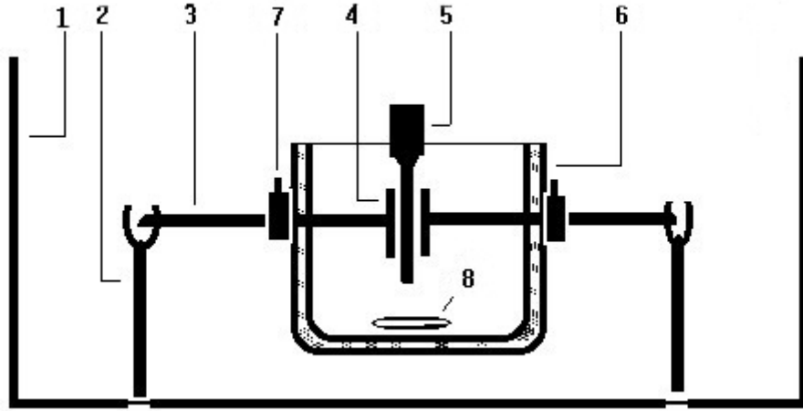
图二 高压舱内布置图
