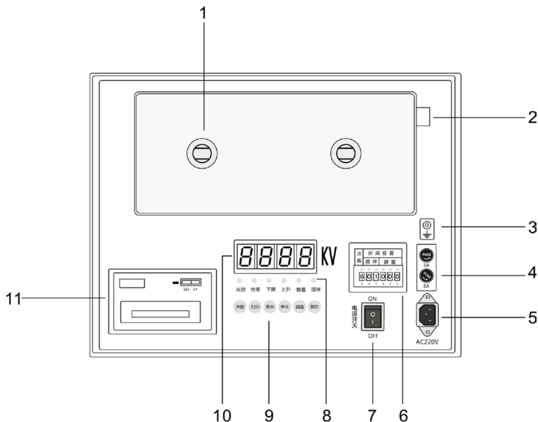
图一 面板示意图
