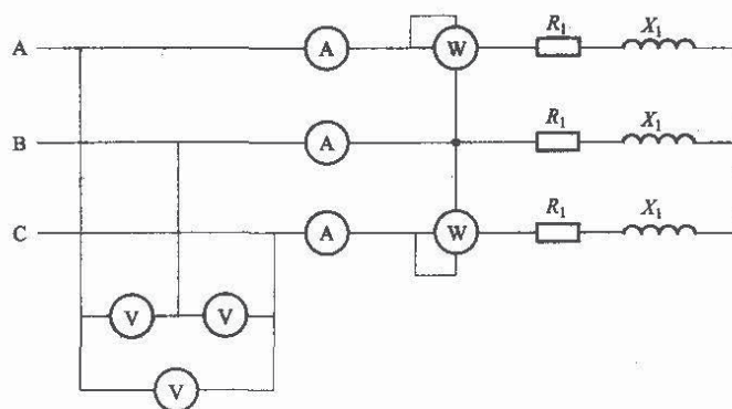
图2 正序阻抗等值集中参数测量电路图
