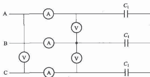
图 4 正序电容等值集中参数测量电路图
